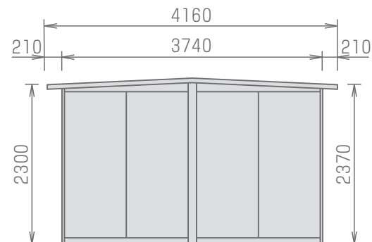
【D立面図】
