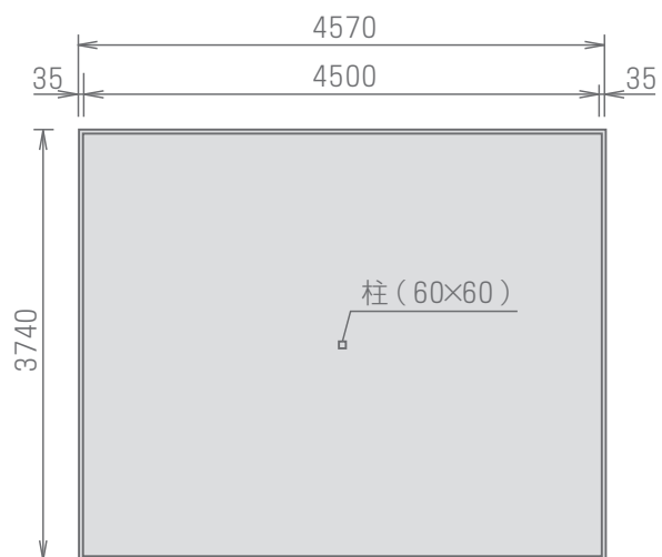
【平面図】
