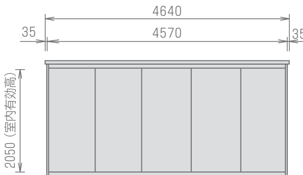
【A立面図】
